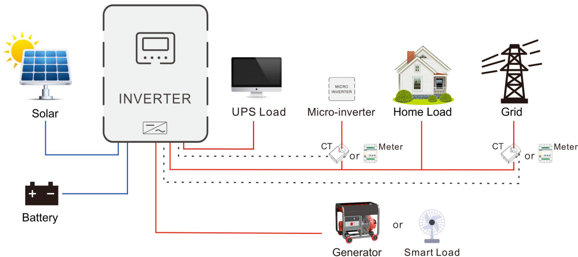
系统接线图二
